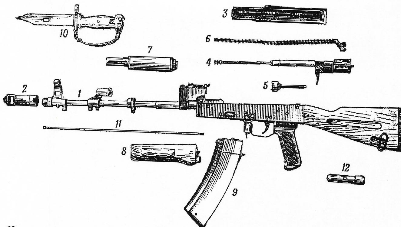
Названия частей и механизмов АК-74м:
